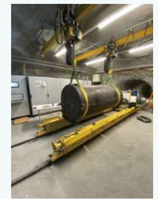
グリムゼル岩盤試験場HotBENT(ペントナイト熱変質試験)試験体 ©Nagra
