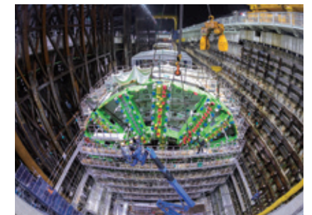
AIシステムを採用する国内最大(外径φ16.1m)のシールドマシン(東京外かく環状道路 本線トンネル(南行)大泉南工事 東京都練馬区)
