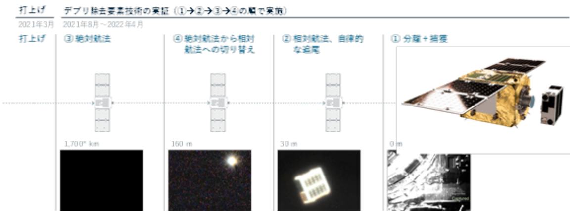
図26 ELSA-dの宇宙実証の内容（*はサービスとクライアントの距離）
