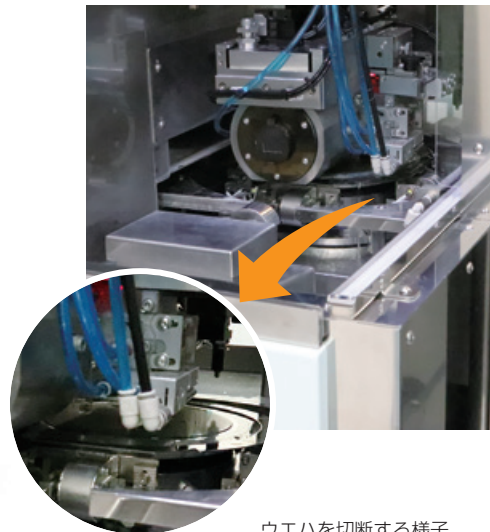
ウエハを切断する様子
