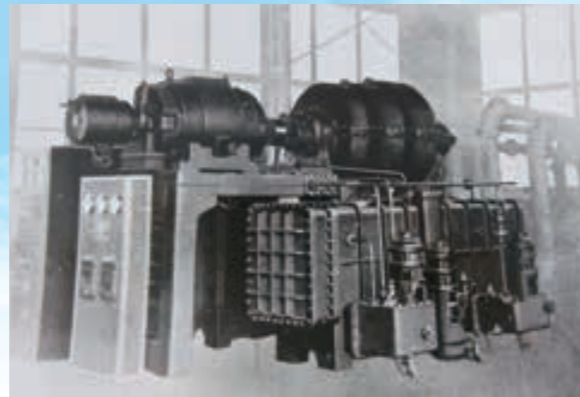
高砂荏原式ターボ冷凍機
