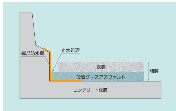
施工断面図
