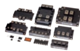
三菱電機(株)製 SiC パワーモジュール
