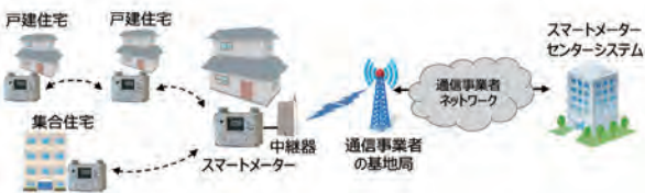
ガススマートメーターシステムの構成
